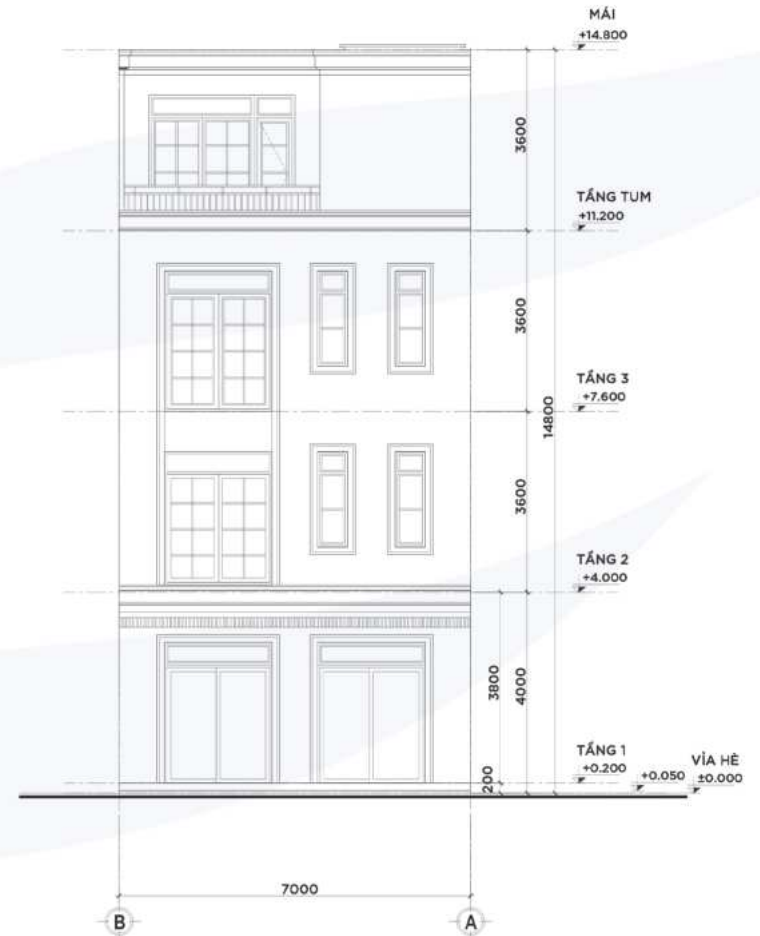
MẶT ĐỨNG TRỰC B-A TỶ LỆ: 1/100
