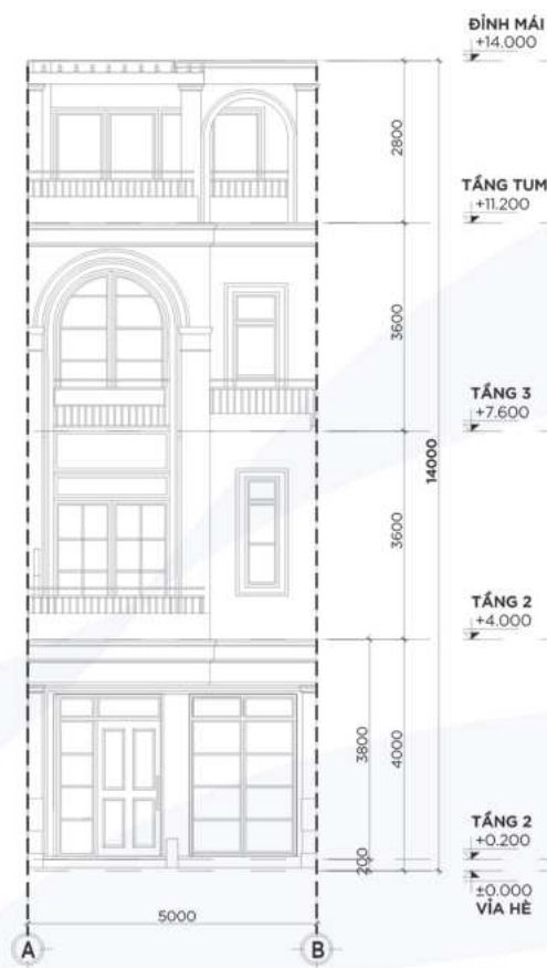
MẶT ĐỨNG TRỰC A-B TỶ LỆ: 1/100
