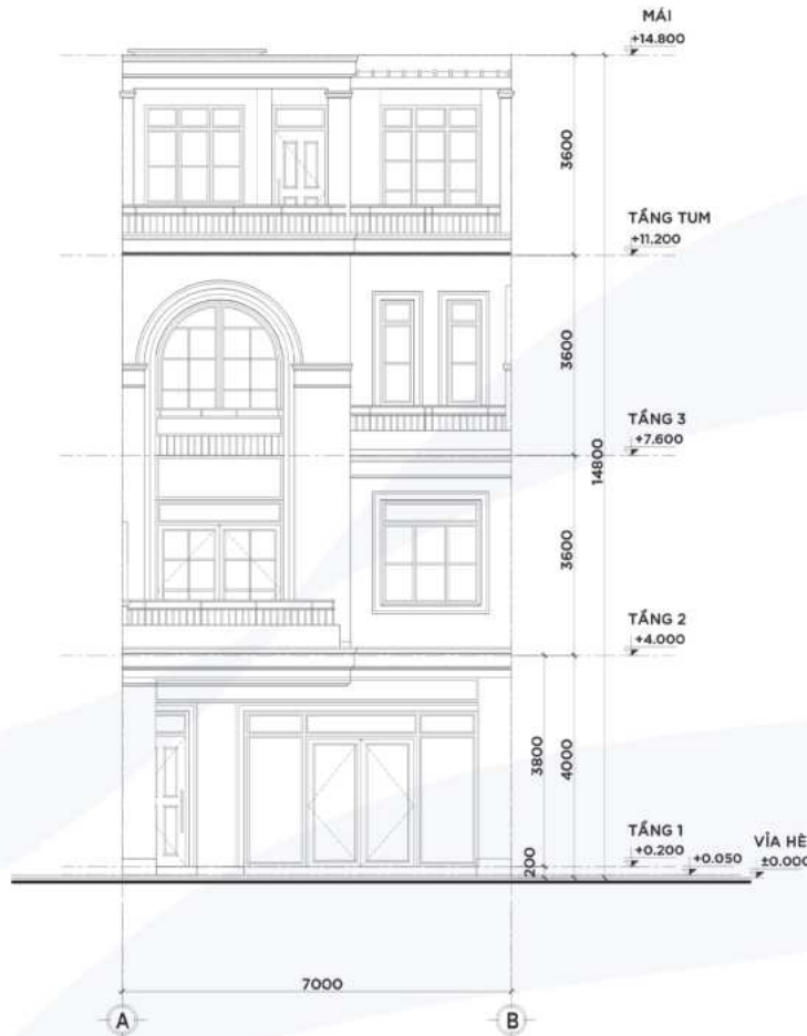
MẶT ĐỨNG TRỰC A-B TỶ LỆ: 1/100
