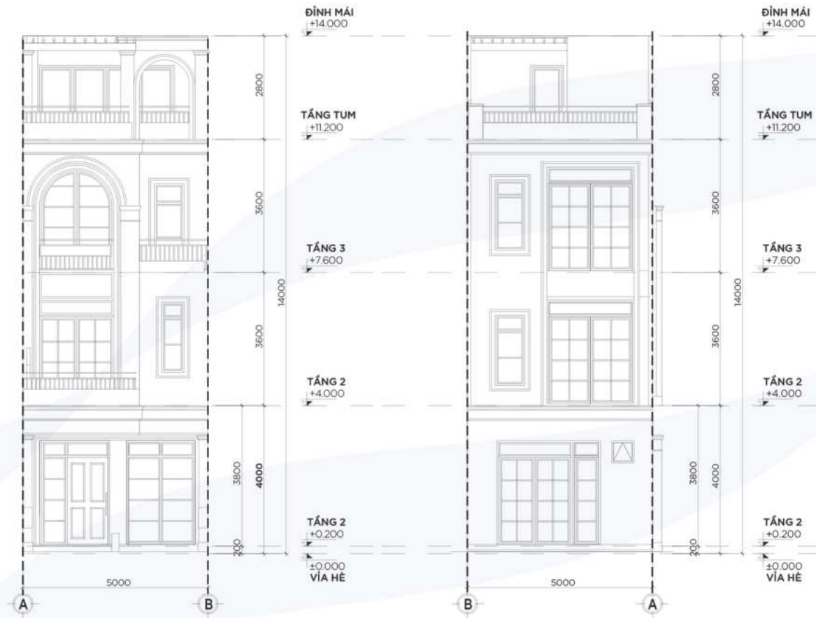
MẶT ĐỨNG TRỰC A-B TỶ LỆ: 1/100
