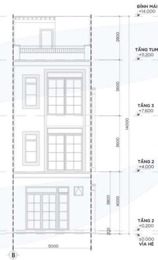
MẶT ĐỨNG TRỰC B-A TỶ LỆ: 1/100
